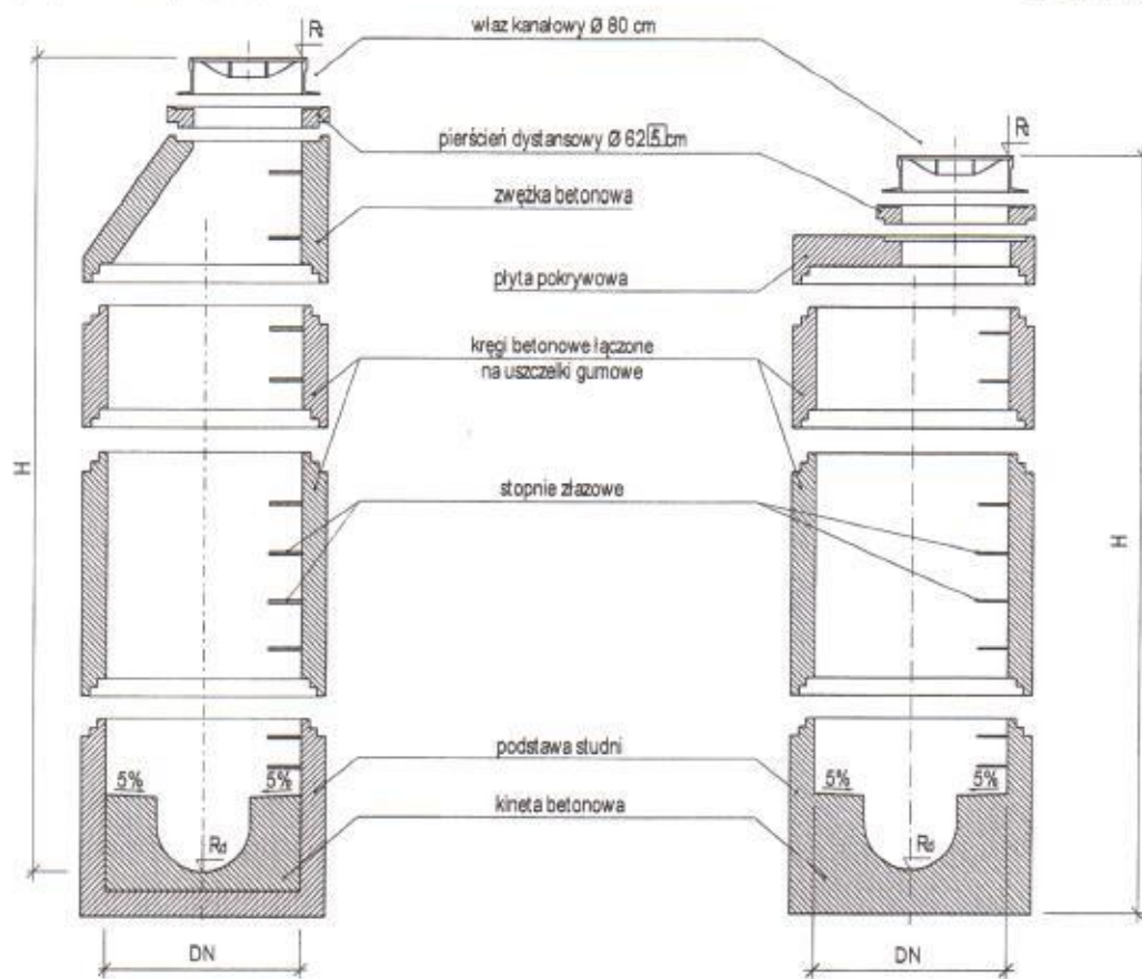
Studzienka kanalizacyjna z płytą pokrywową
