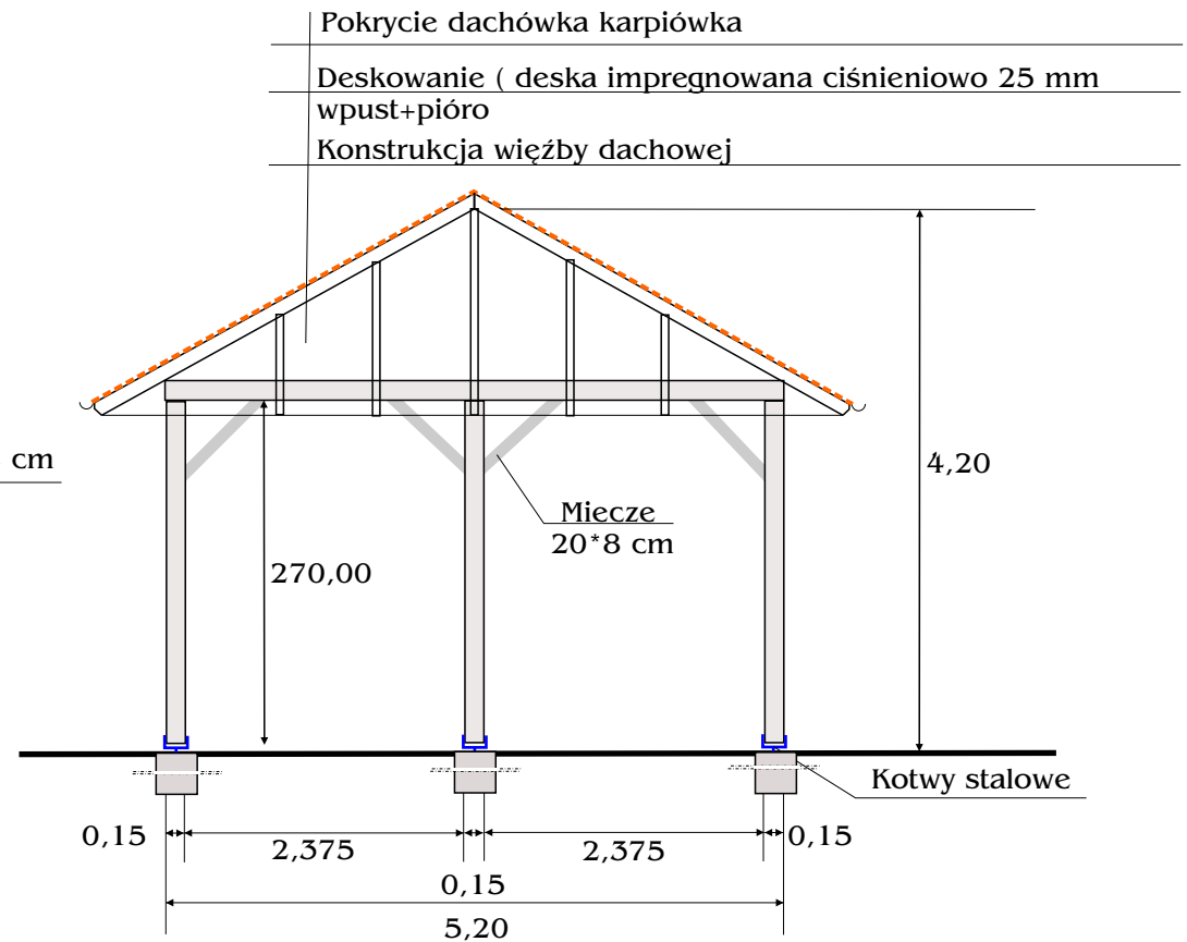
Przekrój pionowy
